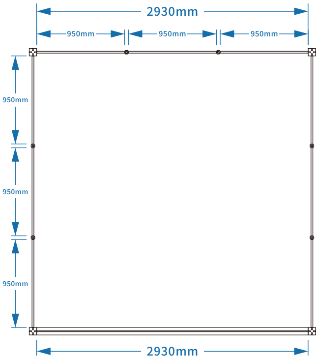
整体平面
