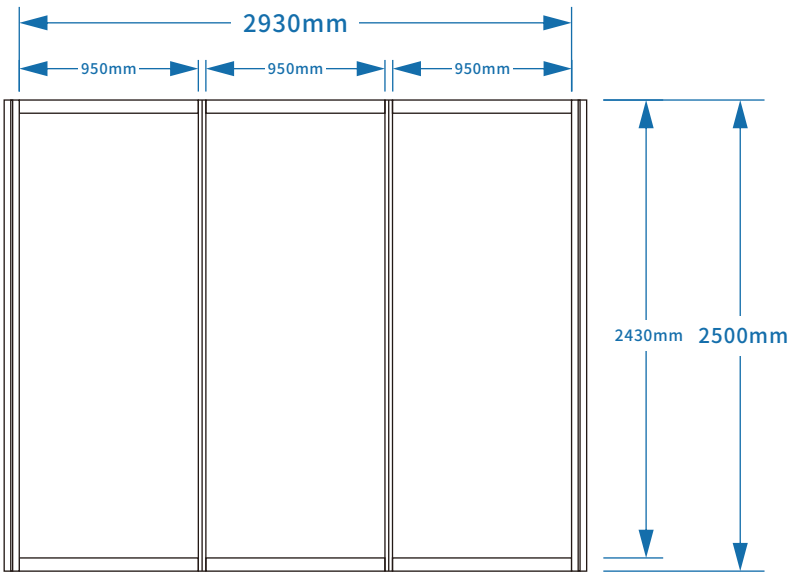
背板立面
