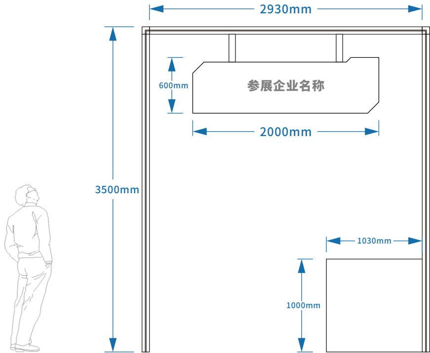
正立面
