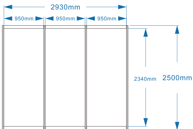
背板立面
