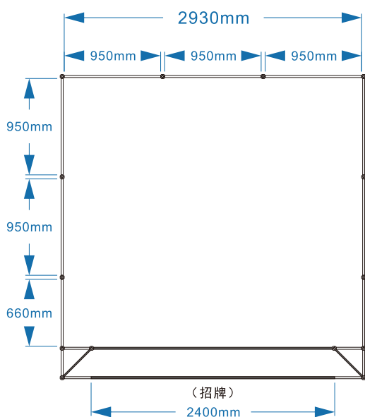
整体平面
