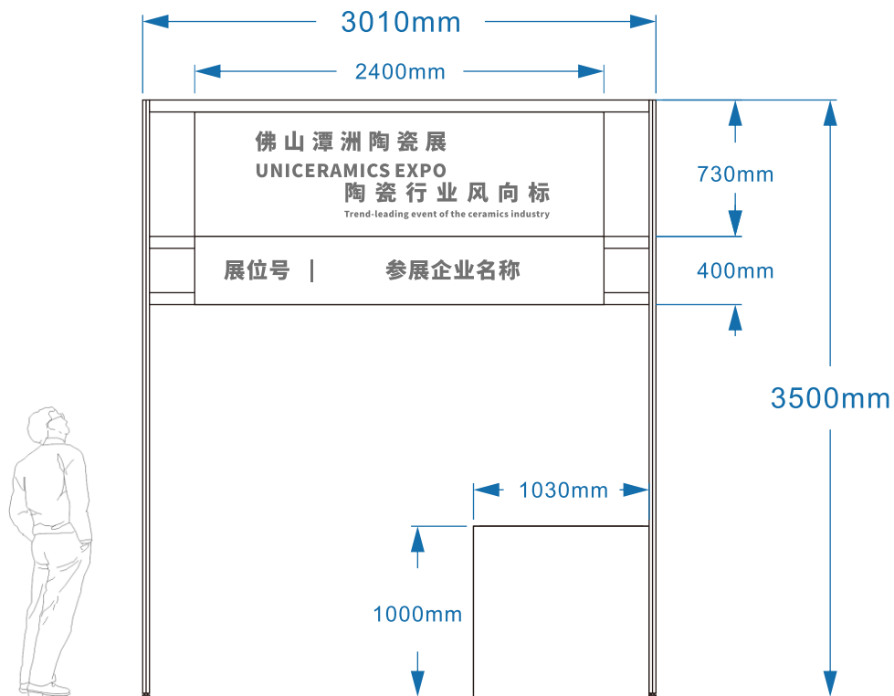
正立面
